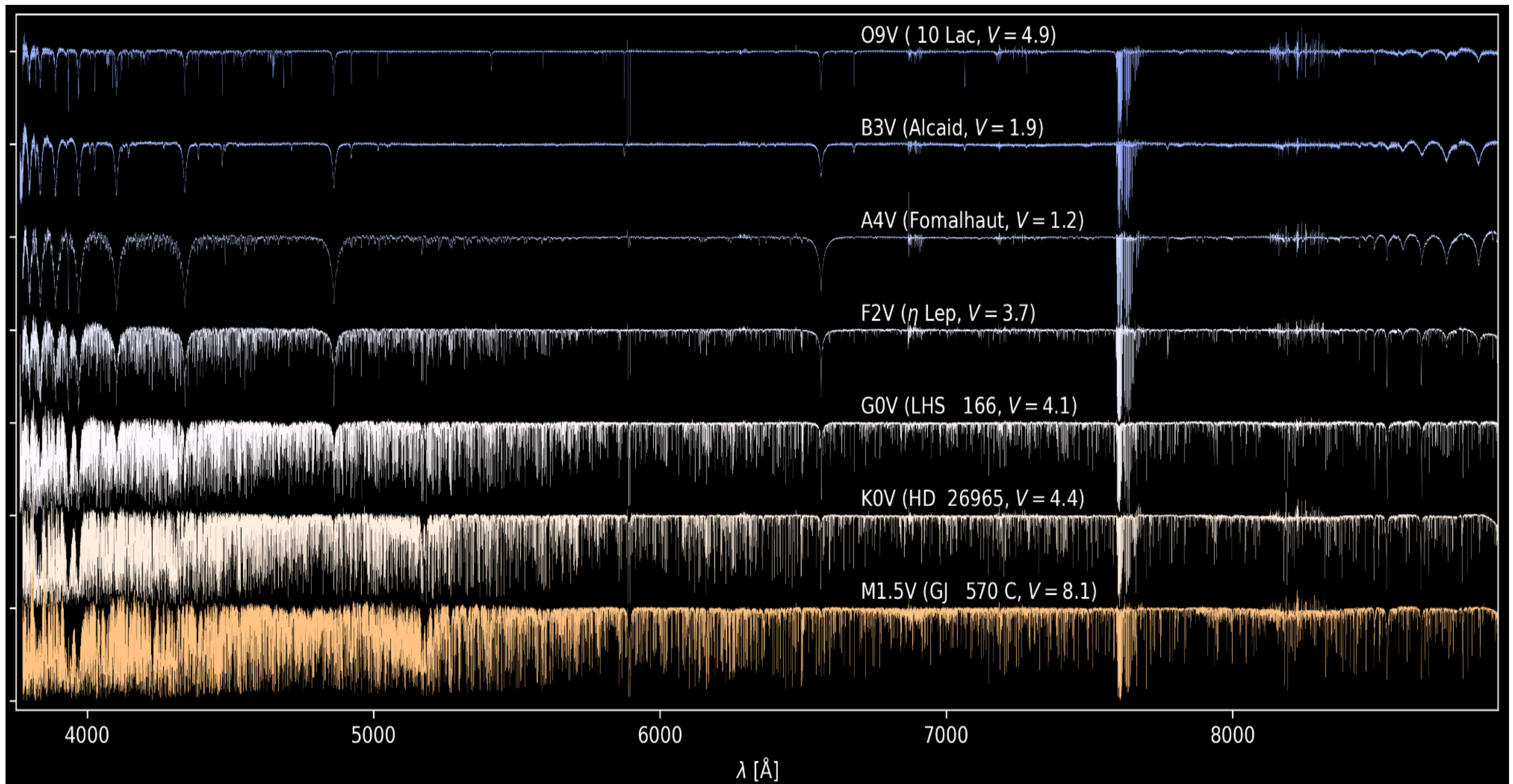
Spectres observés normalisé HERMES d'étoiles de la séquence principale des plus chaudes (type spectral O) aux plus froides (type spectral M).. Crédit: Royer et al. (2024). Genormaliseerde HERMES-spectra van hoofdreekssterren, variërend van de heetste (spectraaltipe O) tot de koelste (spectraaltipe M).. Bron: Royer et al. (2024).
