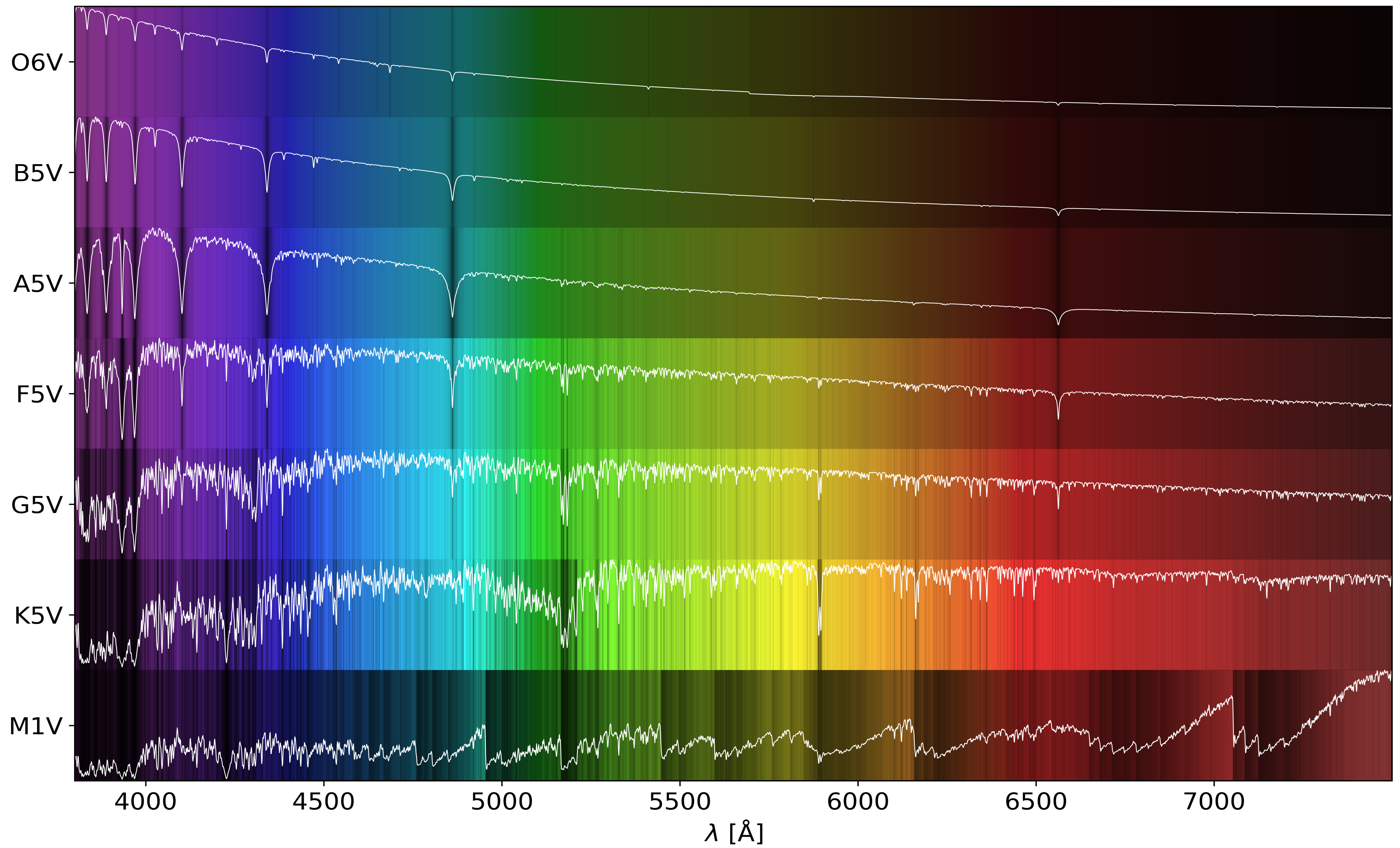
Spectres calculés d'étoiles de la séquence principale des plus chaudes (type spectral O) aux plus froides (type spectral M). Crédit: T. Merle. Berekende spectra van hoofdreekssterren, van de heetste (spectraaltipe O) tot de koelste (spectraaltipe M). Bron: T.Merle.
