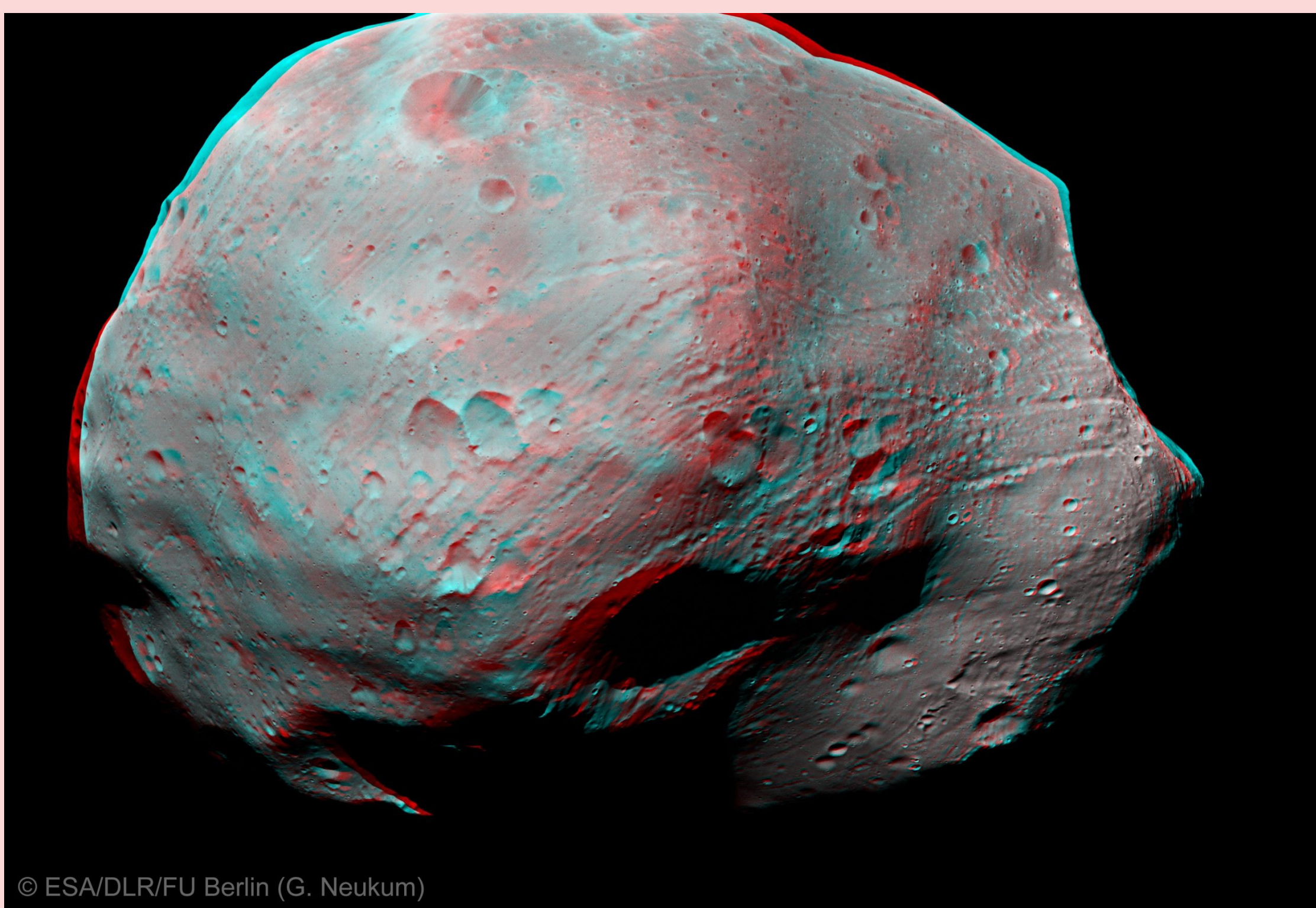
Phobos (lune de mars)
