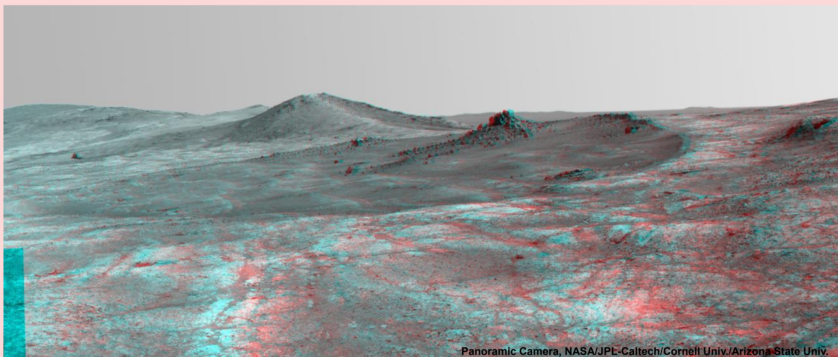
Panorama dans le cratère « Spirit of St. Louis » par le rover Opportunity
