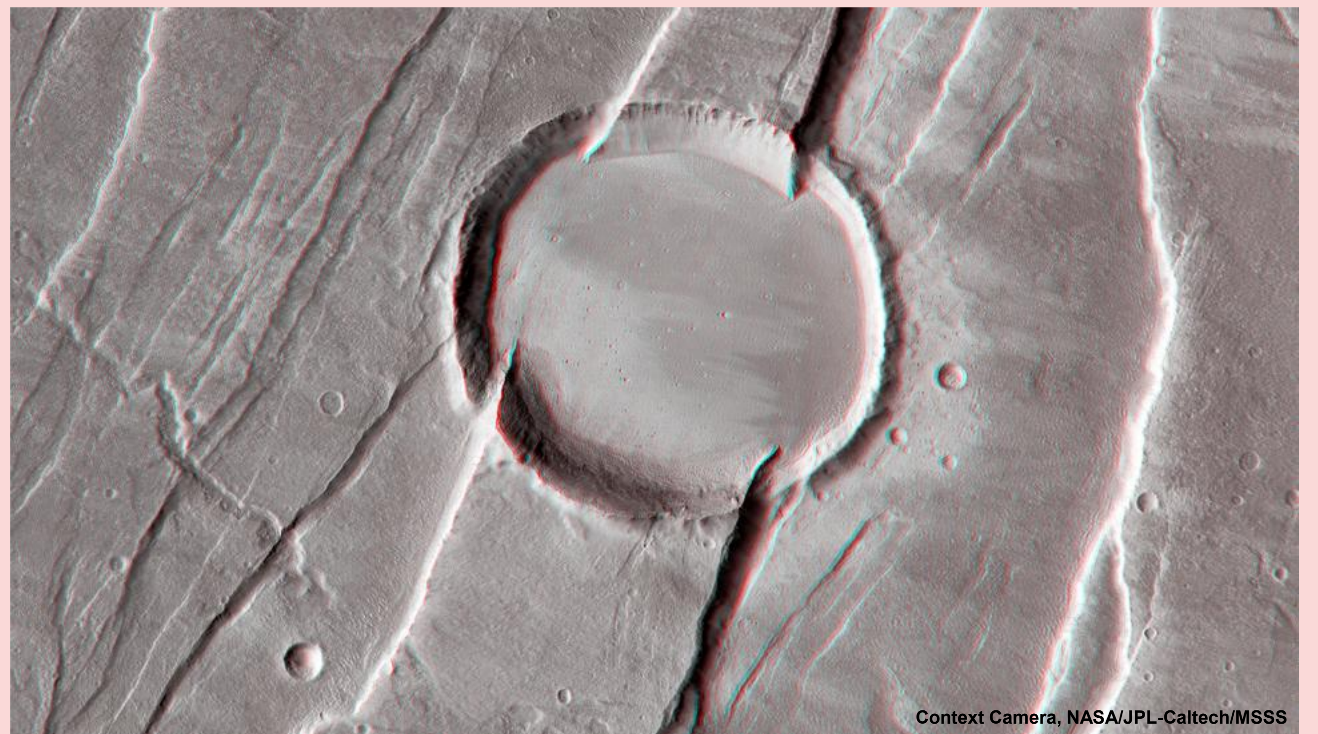
Cratère dans Tantalus Fossae
