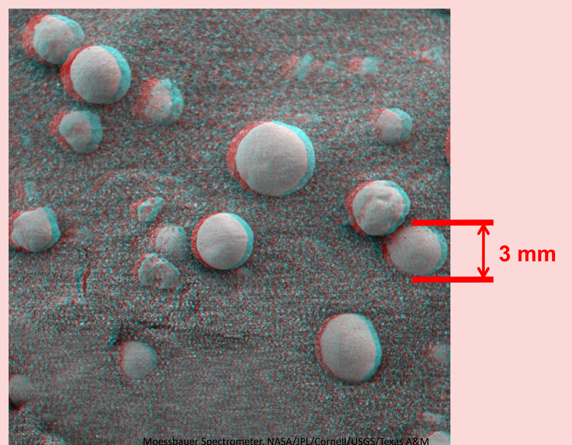
Grains en forme de myrtilles à la surface de Mars
