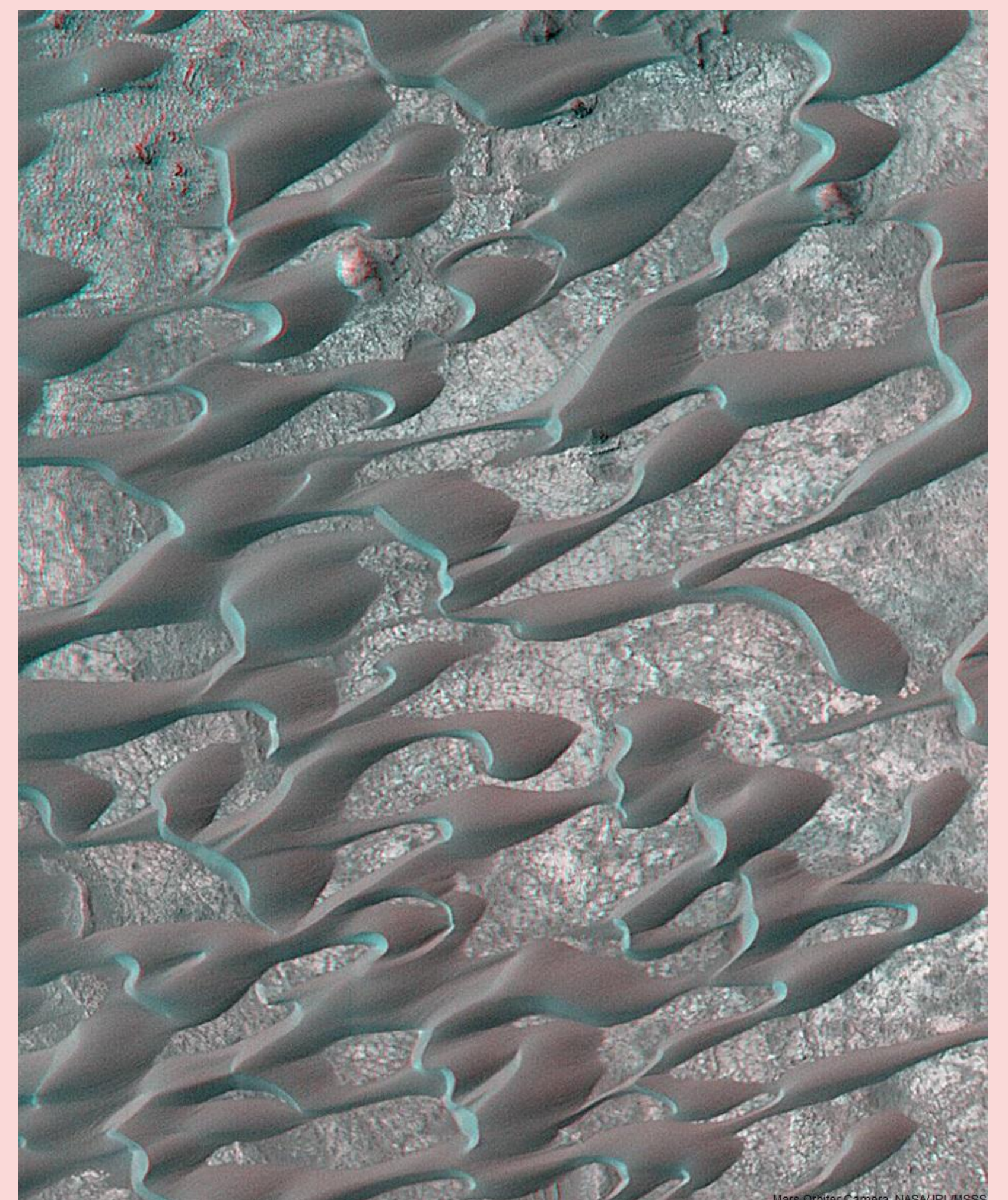
Dunes de sable dans Nili Patera
