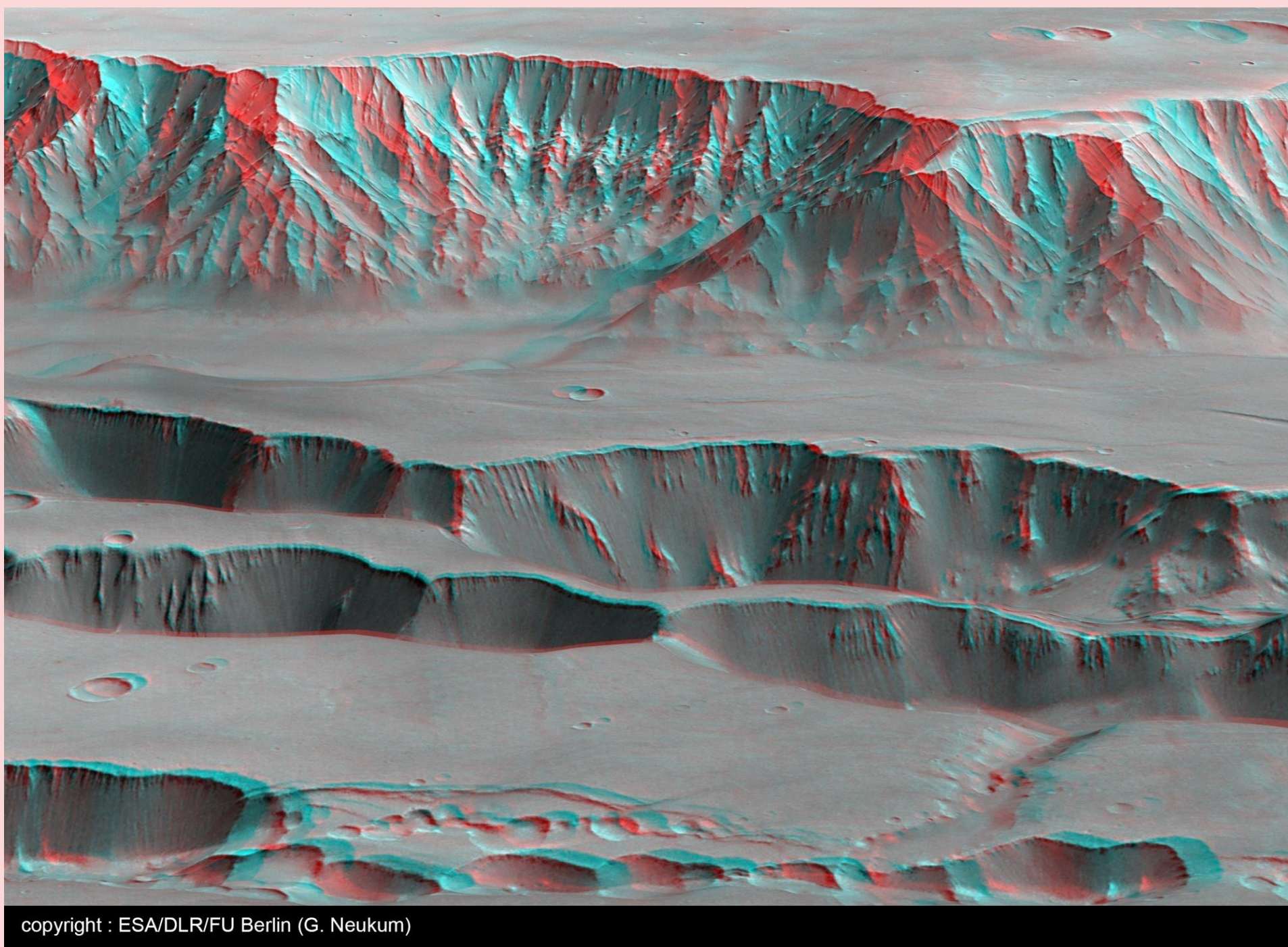
Coprates Chasma, un énorme canyon, dans Valles Marineris
