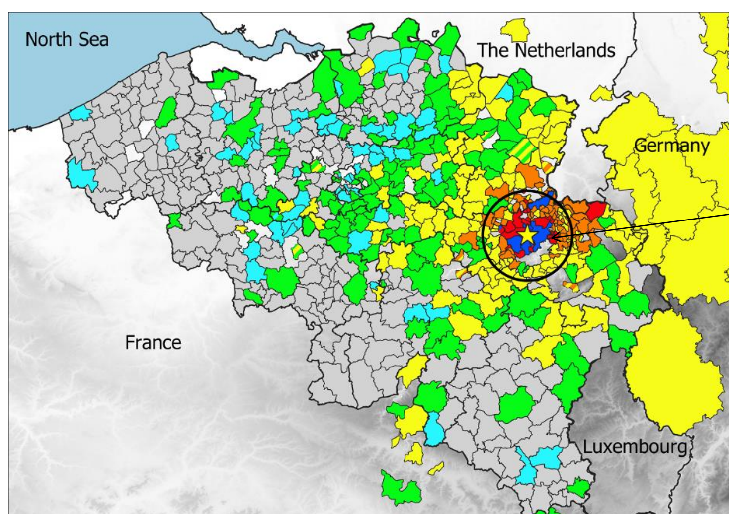
Carte macrosismique de l'événement principal. Crédit : ORB. Makroseismische kaart van de hoofdbeving. Bron: KSB.
