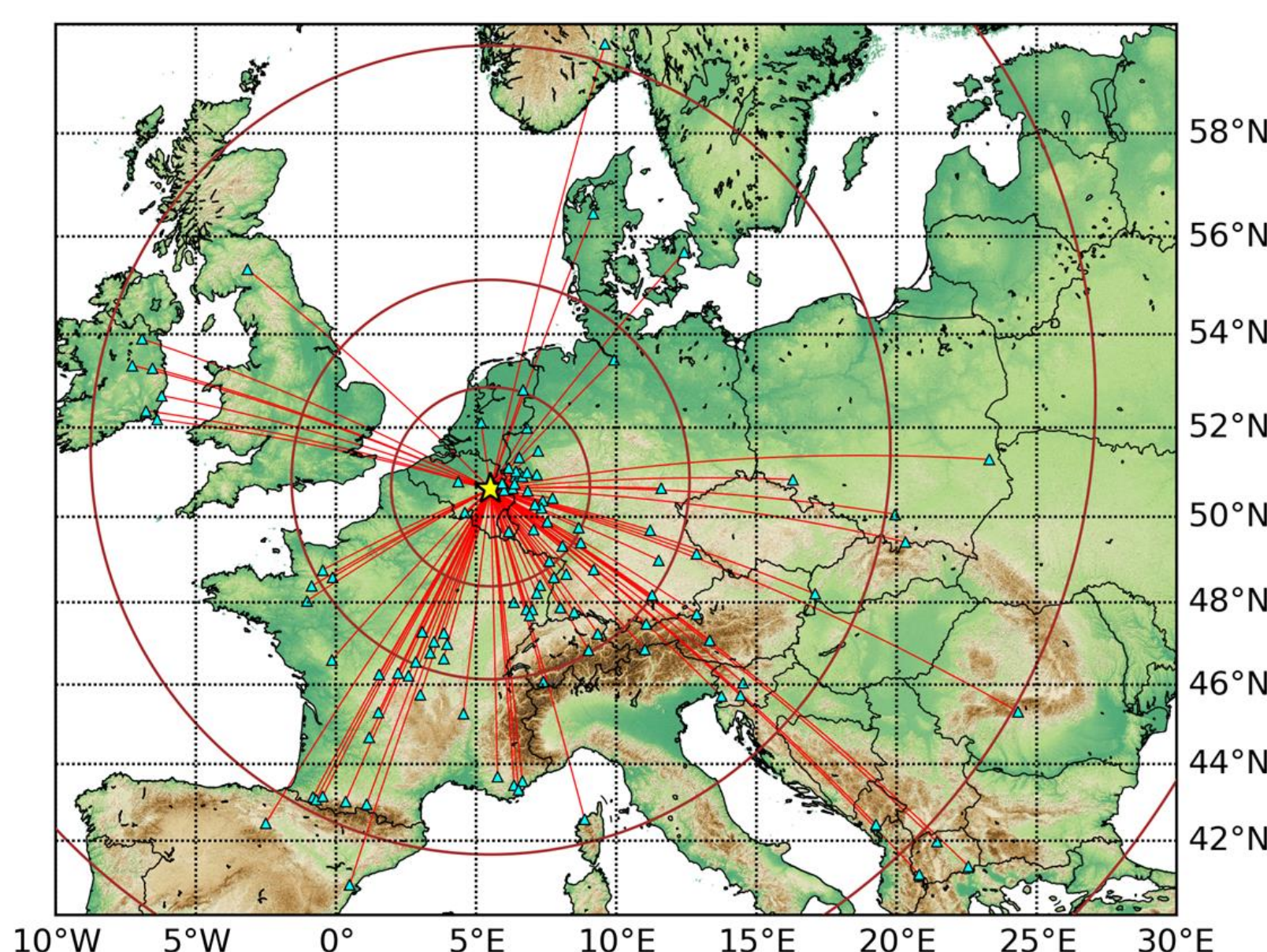
Carte des stations sismiques européennes qui ont enregistré le séisme de Liège. Crédit: ORB. Kaart van de Europese seismische stations die de aardbeving in Luik hebben geregistreerd. Bron: KSB.
