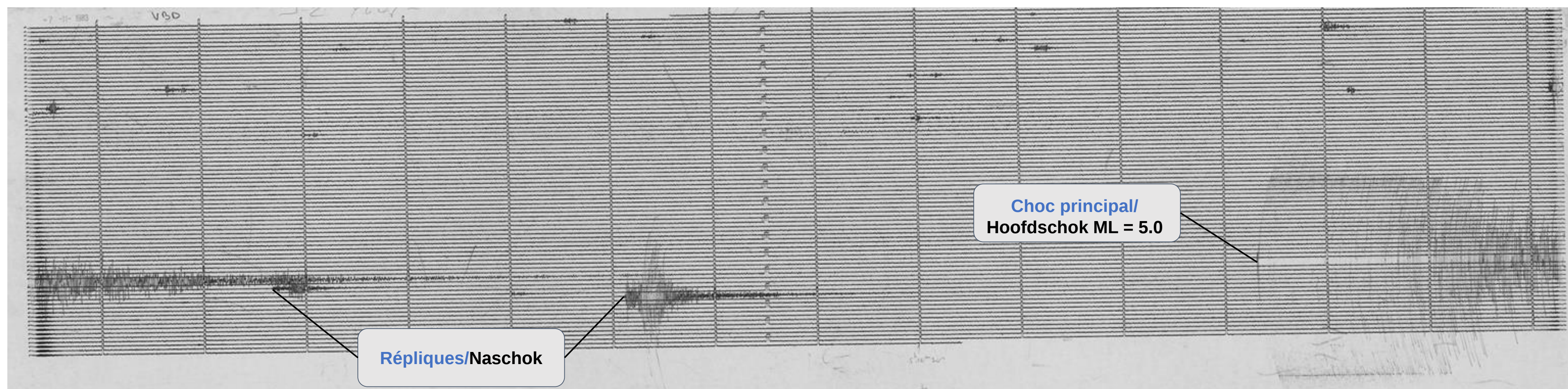
Enregistrements sur papier du tremblement de terre de Liège le 8 novembre 1983 à Dourbes (95 km de l'épicentre). Crédit: ORB. Papieren registraties in Dourbes (95 km van het epicentrum) van de aardbeving in Luik op 8 november 1983. Bron: KSB.
