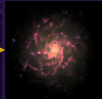
Optical + IR
