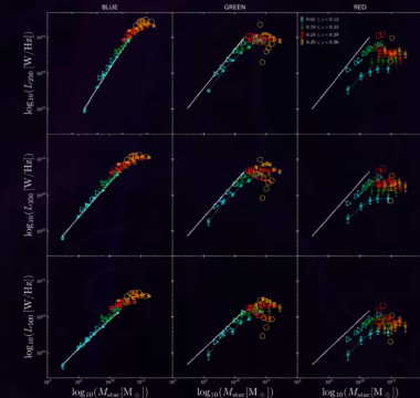
Optical + IR
